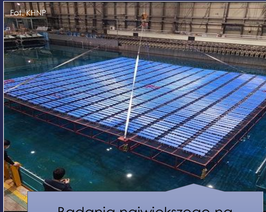
Badania największego na świecie pływającego modelu solarnego w Korei Południowej
